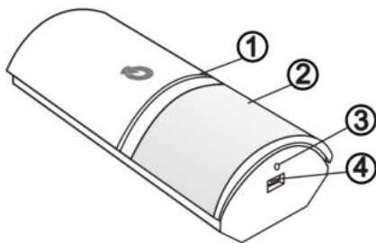
Abbildung 1.: 1 – LED-Anzeigen, 2 – PIR-Linse, 3 – Öffnung für Sicherungsschraube, 4 – Abdeckungslasche
