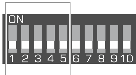
Abb. 4. Schalter zur Einstellung der Adresse, wenn das Funkbasismodul an die Zentrale INTEGRA / INTEGRA Plus angeschlossen ist.
