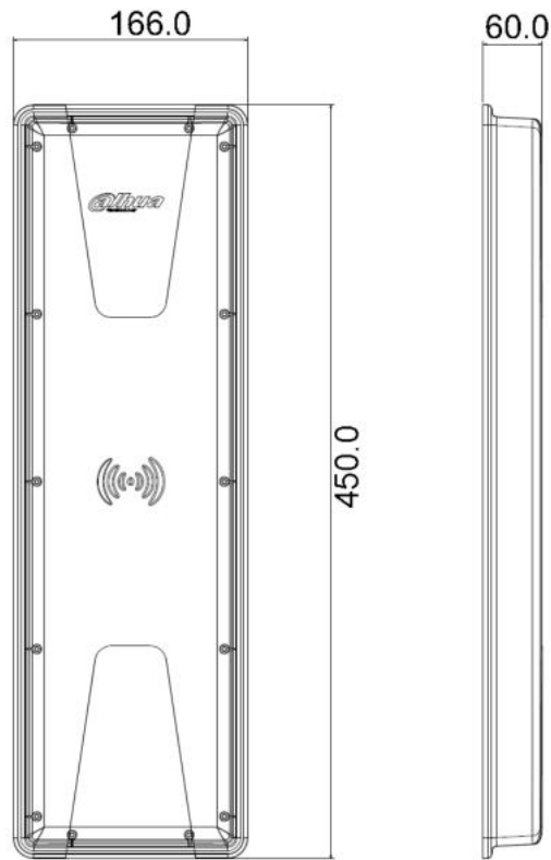
Antenna
