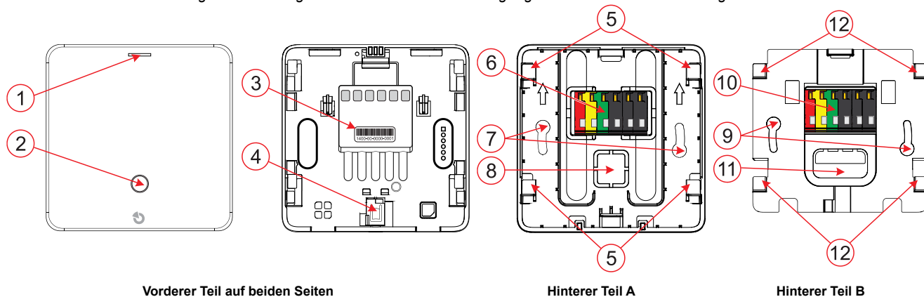
Abb. 1: Beschreibung der einzelnen Teile des Produkts
