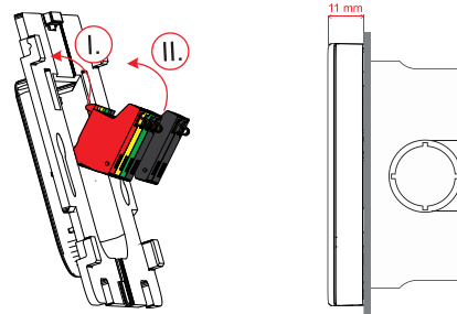
Abb. 3: Illustration einer teilweise versenkten Montage
