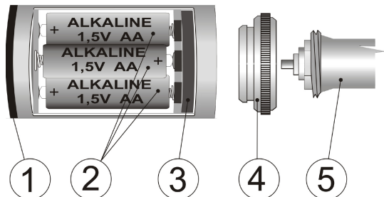
Abb. 1: 1 – Anzeige; 2 – Batterien; 3 – Sicherheitsring; 4 – Adapter; 5 – Heizkörperventil
