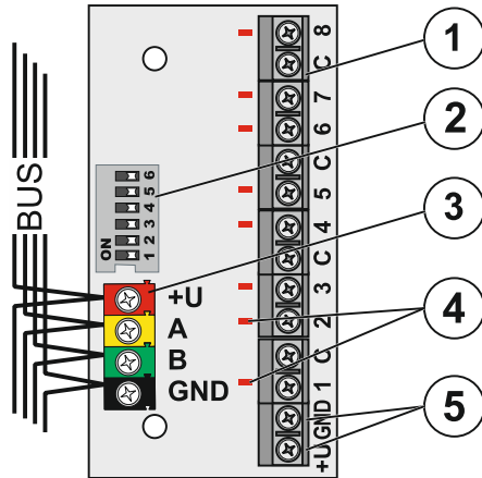
Abbildung: 1 – Ausgangsklemmen; 2 – Konfigurationsumschalter, 3 – Klemmleiste der Sammelleiste; 4 – Signallampen; 5 – Versorgungsanschluss bis 100 mA
