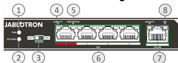
Abbildung 4: Vorderseite des Switch: 1 – Betriebsspannungsanzeige; 2 – PoE-Stromüberlastungsanzeige; 3 – "EXTEND"-Schalter zur Verstärkung der PoE-Stromversorgung, um die maximale LAN-Kabellänge zu verlängern; 4 – Aktivitätsanzeige des LAN-Geräts; 5 – Anzeige für die PoE-Stromversorgung; 6 – RJ-45-Stecker für IP-Kameras mit PoE-Stromversorgung; 7 – RJ-45-Stecker für die Verbindung mit dem Router; 8 – keine Funktion
